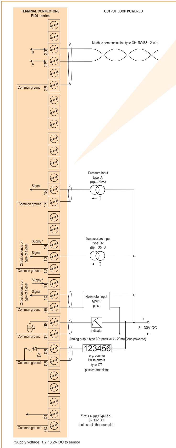
Typical wiring diagram F126-P-AP-CH-EG-IA-OT-(PX)-TA
